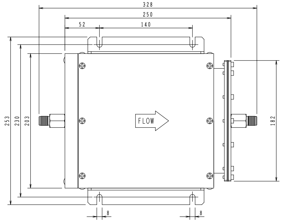
上面図
