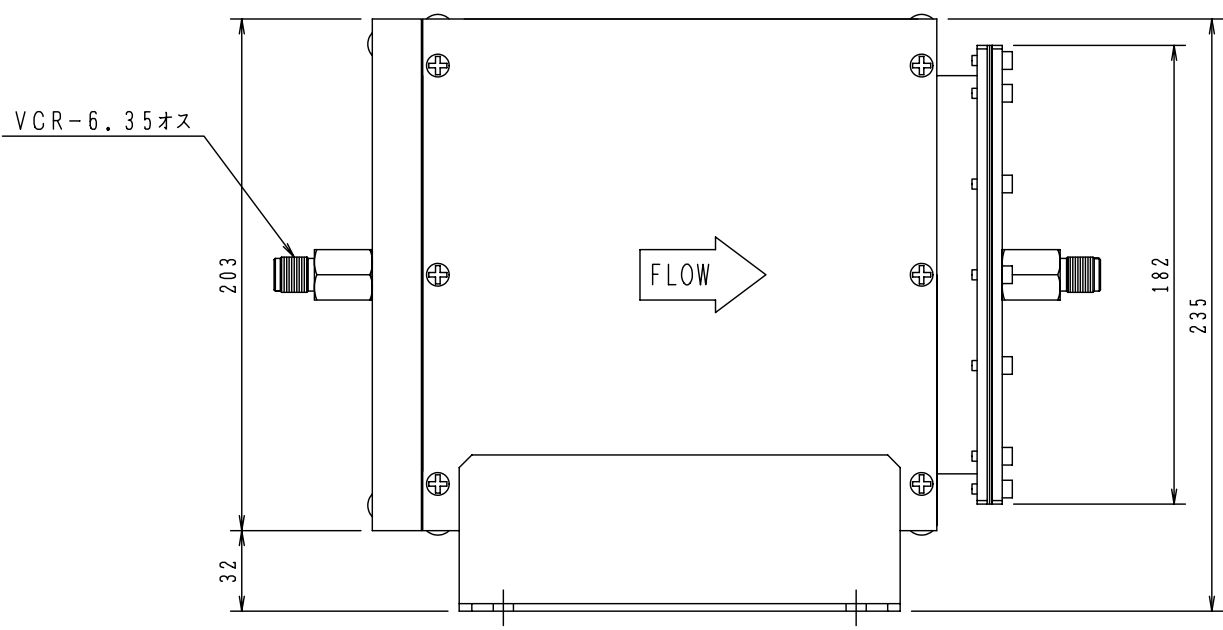
側面図
